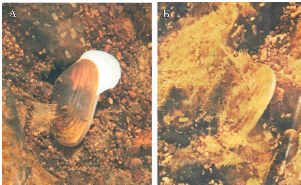
Рис. 34. Экземпляры Middendorffinaia mongolica (Middendorff, 1851) в р. Комаровка, приклеенные ловчими сетями личинок ручейников Stenopsyche marmorata Navás, 1920 к валунам (А – 29.10.2021; Б – 19.11.2021). Фото автора
