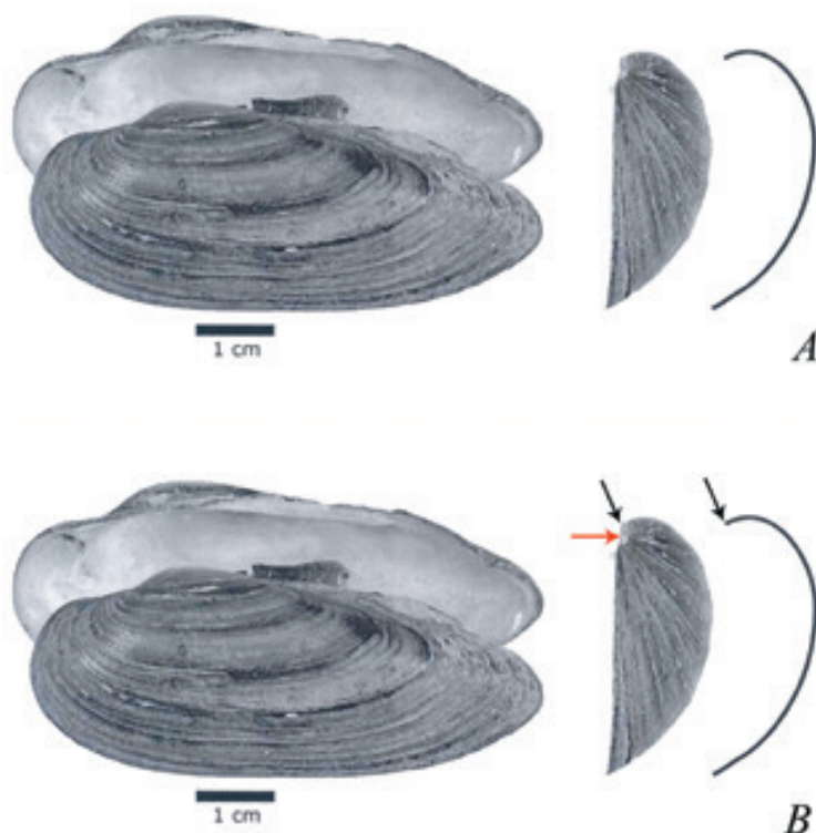
Рис. 16. Интерпретция в работе Графа [Graf, 2007] схемы зарисовки фронтального контура створки относительно оси обзора со ссылкой на работу Шикова и Затравкина [Shikov, Zatravkin, 1991] ( A ); тот же рисунок: черными стрелками показана точка, от которой, по мнению автора, разворачивается спираль контура; на самом деле начальная точка разворачивания спирали контура расположена ниже, в точке схождения линий роста (показано красной стрелкой) ( B )
