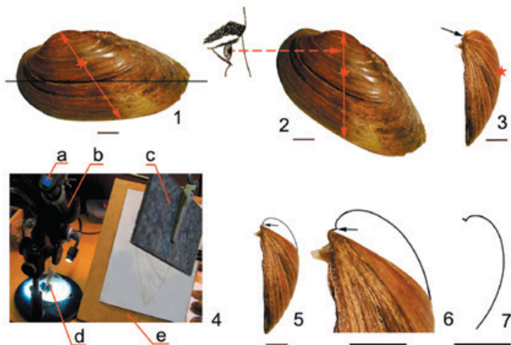
Рис. 12. Определение максимально выпуклого контура левой створки Unio модифицированным компараторным методом: 1 – вид створки сбоку; 2 – положение створки для прорисовки МВК; 3 – вид спереди в позиции просмотра МВК; 4 – стереоскопический бинокулярный микроскоп MBS-2 с прикрепленным рисовальным аппаратом Аббе (а – светоделительная призма, b – микроскоп, c – зеркало, d – раковина Bivalvia, установленная на пластилине для просмотра, e – подставка с листом бумаги для зарисовки контуров); 5 – прорисованный участок верхней трети МВК; 6 – то же при большем увеличении; 7 – итоговый рисунок МВК. Сплошной красной линией на створках показано боковое положение линии МВК, пунктирной линией – направление просмотра для зарисовки МВК, звездочкой отмечена наиболее выступающая точка боковой поверхности створки, черными стрелками – центр спирали (точка, из которой разворачивается спиралеобразный контур). Масштаб 1 см
