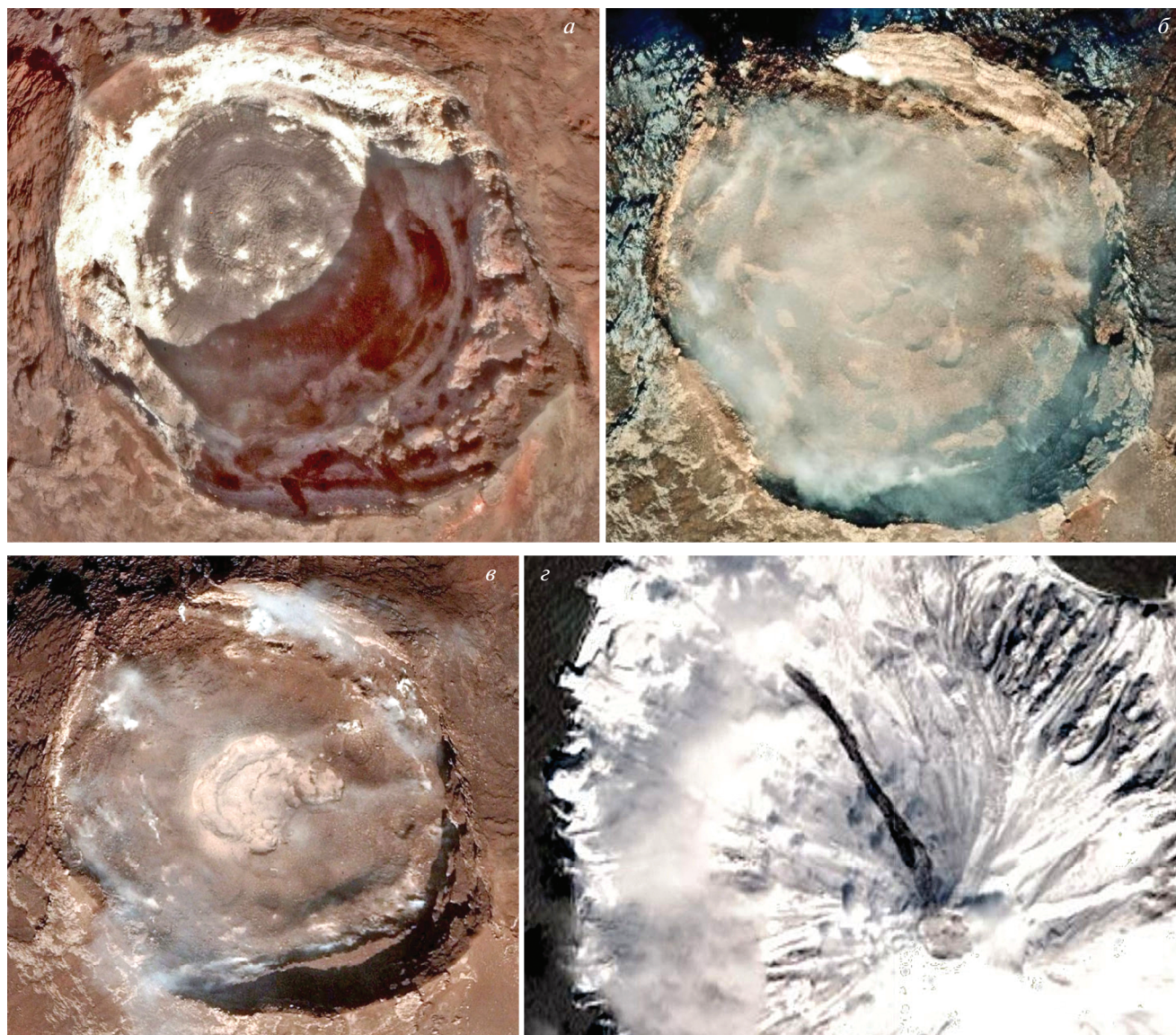
Рис. 3. Кратер вулкана Пик Сарычева: а – 31.08.2016, ИСЗ WorldView-2; б – 05.10.2018, ИСЗ WorldView-4; в – 07.09.2019, ИСЗ GeoEye-1; г – кратер и лавовый поток на склоне, 16.04.2021, ИСЗ WorldView-2.
