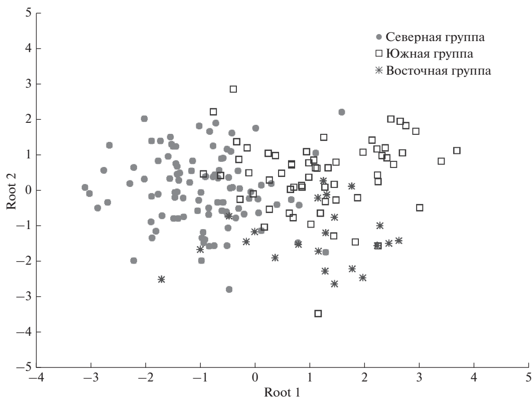
Рис. 5. Распределение экземпляров пищух по размерным характеристикам p_3 .
