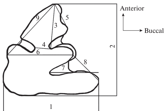
Рис. 1. Схема промеров р 3 северной пищухи Ochotona hyperborea . Пояснения в тексте.
