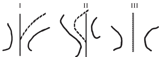
Рис. 2. Схема положения перешейка относительно вершины антероконида: I — изогнутый перешеек, II — S-образный перешеек, III — прямой перешеек. Пунктирная линия показывает направление перешейка относительно вершины антероконида.
