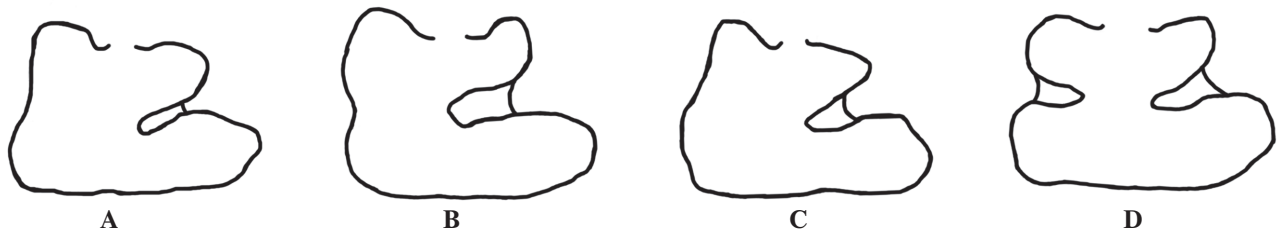
Рис. 4. Форма постероконида. Пояснения в тексте.
