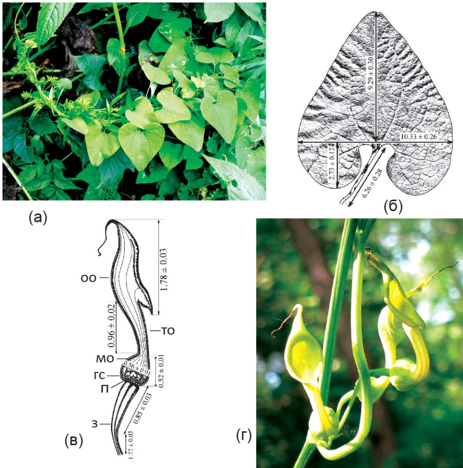
Рис. 16. Внешний вид Aristolochia contorta : (а) – лиана, (б) – лист, (в) и (г) – цветок (фото О.В. Наконечной): гс – гиностемий, з – завязь, мо – мешочек околоцветника, оо – отгиб околоцветника, п – пыльники, то – трубка околоцветника.
