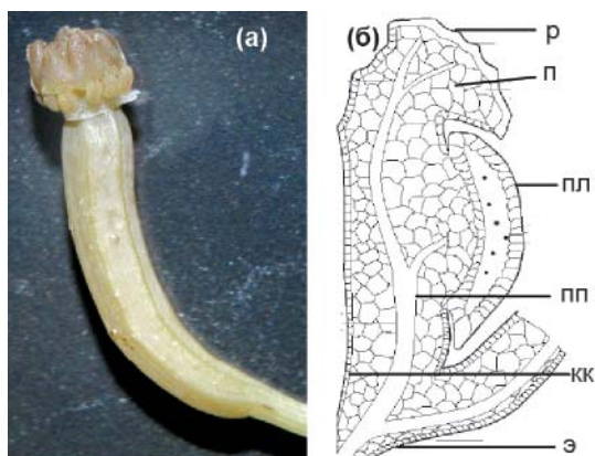
Рис. 24. Строение гинецея и андрогцея Aristolochia contorta : (а) – внешний вид (фото О.В. Наконечной); (б) – схема продольного строения рыльца и столбика.
