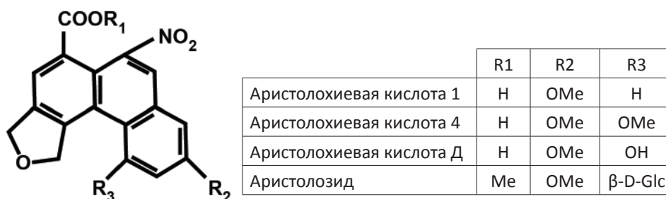
Рис. 43. Структурные формулы аristolохиевых кислот, содержащихся в растениях кирказона Aristolochia manshuriensis .
