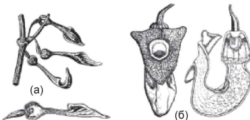
Рис. 5. Цветки представителей рода Aristolochia : (а) — A. clematitis (Кернер, 1902) и (б) — A. macrophylla (Cronquist, 1981).
