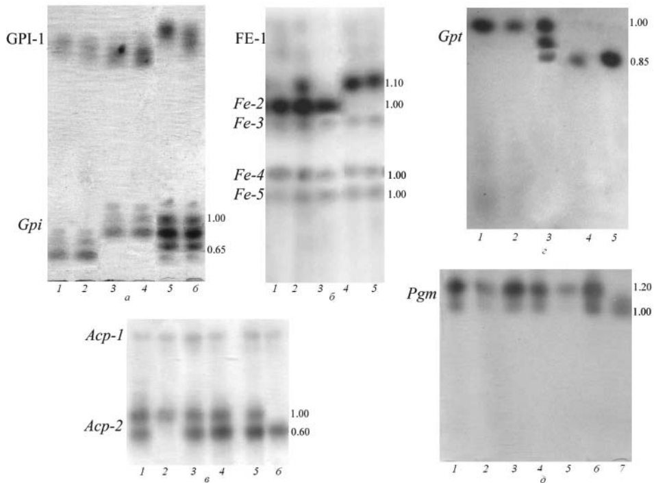
Рис. 35. Электрофореграммы полиморфных ферментов из листьев Aristolochia manshuriensis :
