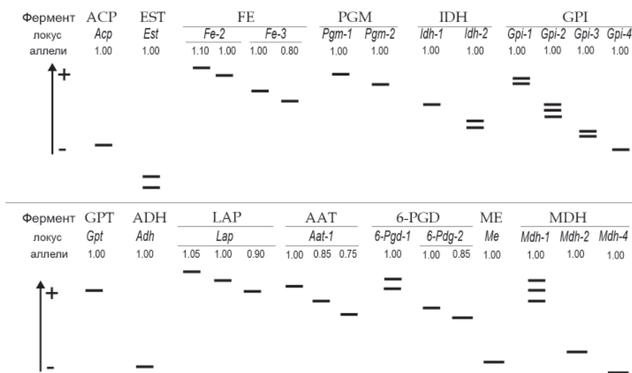
Рис. 40. Схематическое изображение некоторых электрофоретических вариантов ферментов в листьях Aristolochia contorta .
