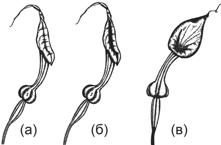
Рис. 30. Схема раскрытия венчиковидного околоцветника Aristolochia contorta .
