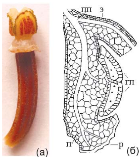
Рис. 21. Строение гинецея и андроцея Aristolochia manshuriensis :
