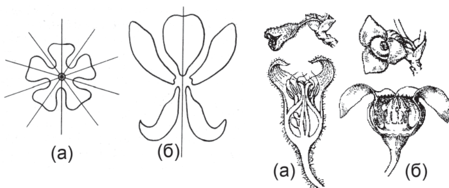
Рис. 3. Симметрия цветка: (а) — актиноморфный, или правильный цветок; (б) — зигоморфный, или неправильный цветок (Яблоков, Челомбитько, 1990).
