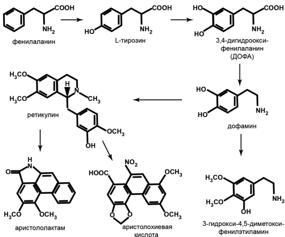
Рис. 45. Биосинтез вторичных метаболитов в клеточной культуре Aristolochia manshuriensis (штамм A2s).
