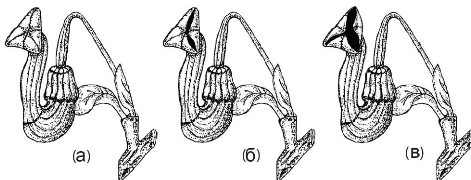
Рис. 27. Схема раскрывания венчиковидного околоцветника Aristolochia manshuriensis .
