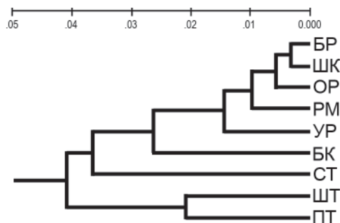
Рис. 42. UPGMA-дендрограмма сходства популяций Aristolochia contorta , построенная на основе коэффициентов генетической дистанции Нея ( D_N ).
