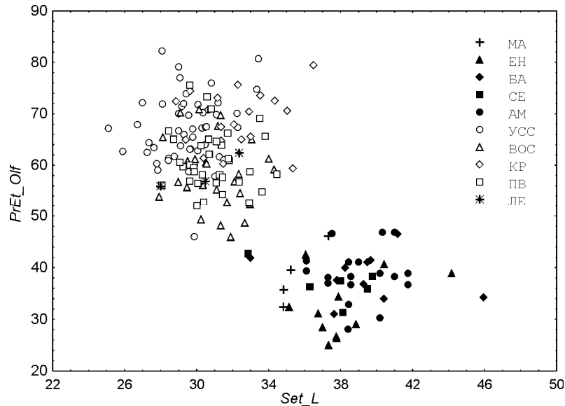
Рис. 3. Распределение особей тупорылых и острорылых (залитые символы) ленок в пространстве двух остеологических индексов. Расшифровку обозначения выборок см. в примечании к табл. 2
