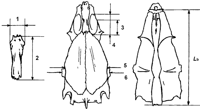
Рис. 2. Схема промеров супраэтмоида (supraethmoideum) и черепа ленок. Все измерения проводились при помощи штангенциркуля. Промеры были использованы для составления следующих индексов: SethW=1/2 (отношение промеров 1 и 2); Pr\_Eth = 3/L_b ; Olf\_cav = 4/L_b ; PrEt\_Olf=3/4 ; PrEt\_Set=3/2 ; Pr\_Sph=(6-5)/L_b ; PrSp\_Set=(6-5)/2 ; Set\_L=2/L_b . L_b – длина основания черепа
